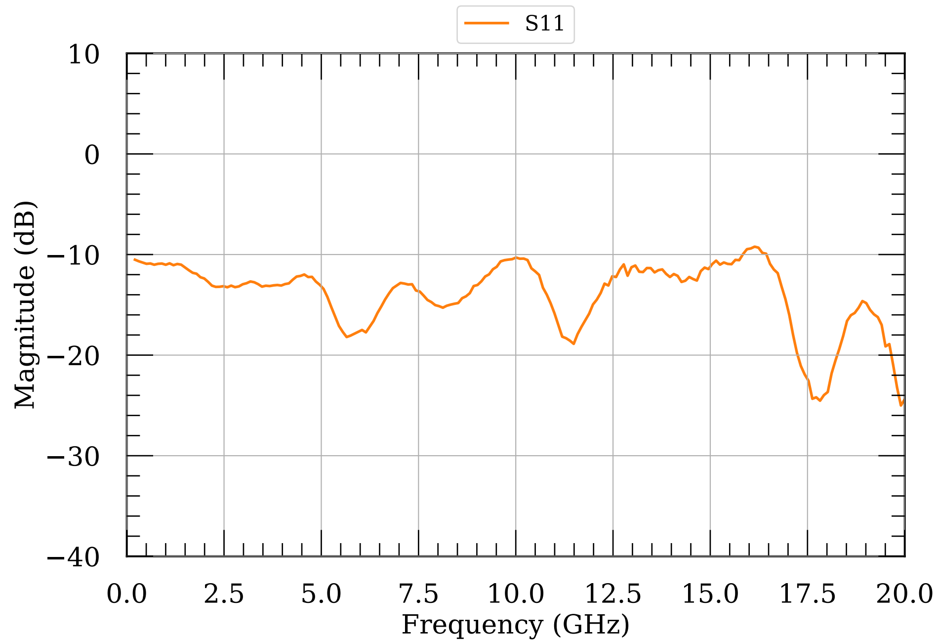
LNA S-params module016
